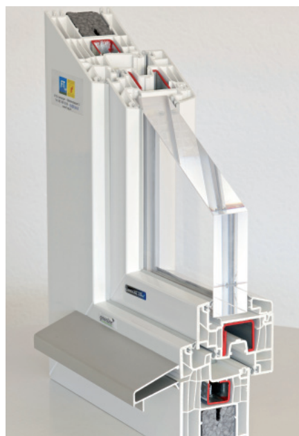
Das Fenstermodell «InVitra» vereint Design, Funktion, Bauphysik und Umweltschutz.
